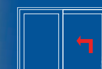
Vierdelig element met twee hefschuifvleugels en twee vaste beglazingen
