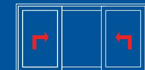
Driedelig element met twee hefschuifvleugels en vaste beglazing
